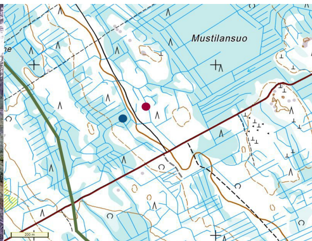
Kartta 6. Mustilansuo.
