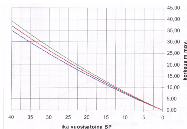
Kartta 4. Kalibroitu rannansiirtymäkäyrä lin alueelle (Okkonen 2003, liite 9 viitteineen).
