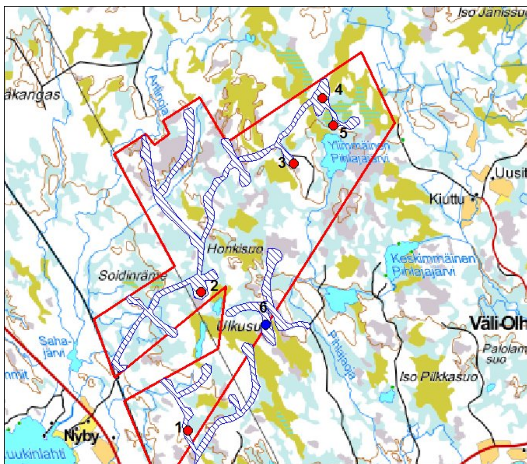
Kartta 6. Yleiskartta, kohteet 1-6 hankealueella. Numerot viittaavat kohdenumerointiin raportissa. Tarkastetut alueet merkitty sinisellä vinoviivituksella. Maanmittauslaitoksen maastokarttarasteri 1:50 000, 10/2015.
