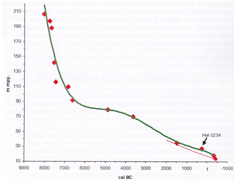
Kartta 3. Kalibroitu rannansiirtymäkäyrä Perämeren pohjukan alueelle (Okkonen 2003, 91 viitteineen).
